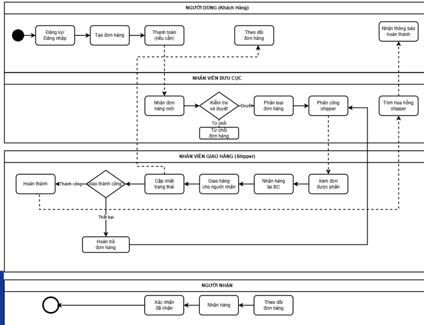
SƠ ĐỒ NGHIỆP VỤ - HỆ THỐNG QUẢN LÝ GIAO HÀNG HPship
